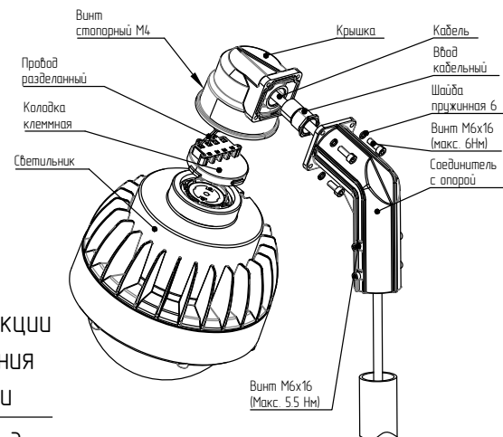
Светильник, взрыв-схема
