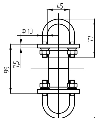
Поворотный механизм
