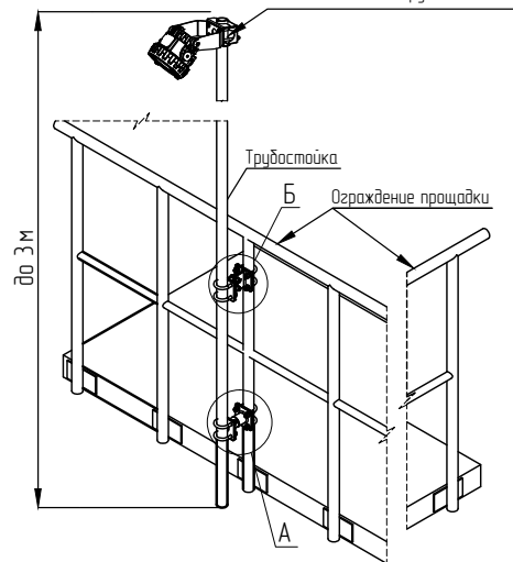
Светильник FLINT с креплением на опору
