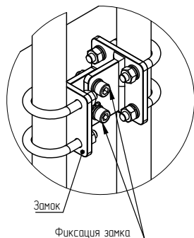
Фиксация замка
