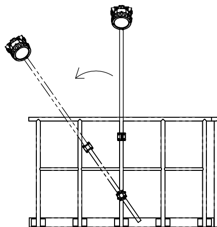
Поворотное устройство для трубостойки
