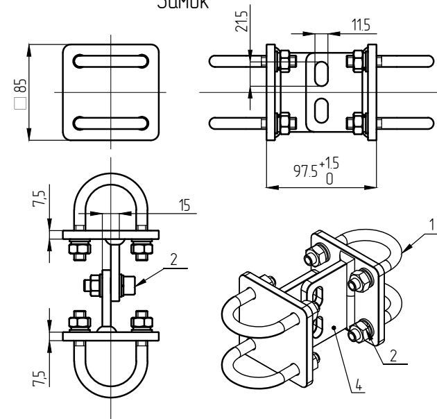
Замок
